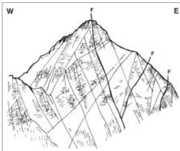
FIG. 9-A. Definición de la forma del K2. La pirámide es modelada según los cruces de sus fallas (F), su red de fracturas y el bandeado del roqueado. Su disposición general realizada en el Karakorum se muestra en la figura 4. (Esquema a partir de Gansser, 1964).
