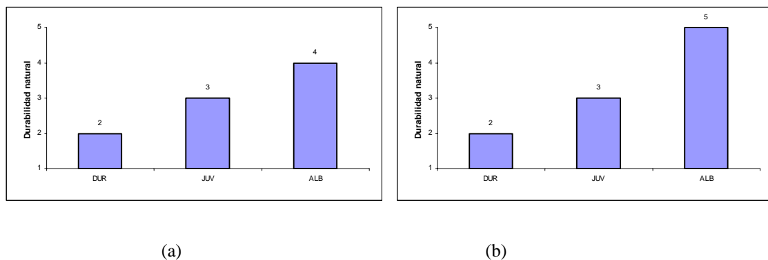
Fig. 1.- Valores medios de la durabilidad natural obtenida para albura (ALB), duramen (DUR) y madera juvenil (JUV) con (a) Trametes versicolor y (b) Chaetomium globosum .
