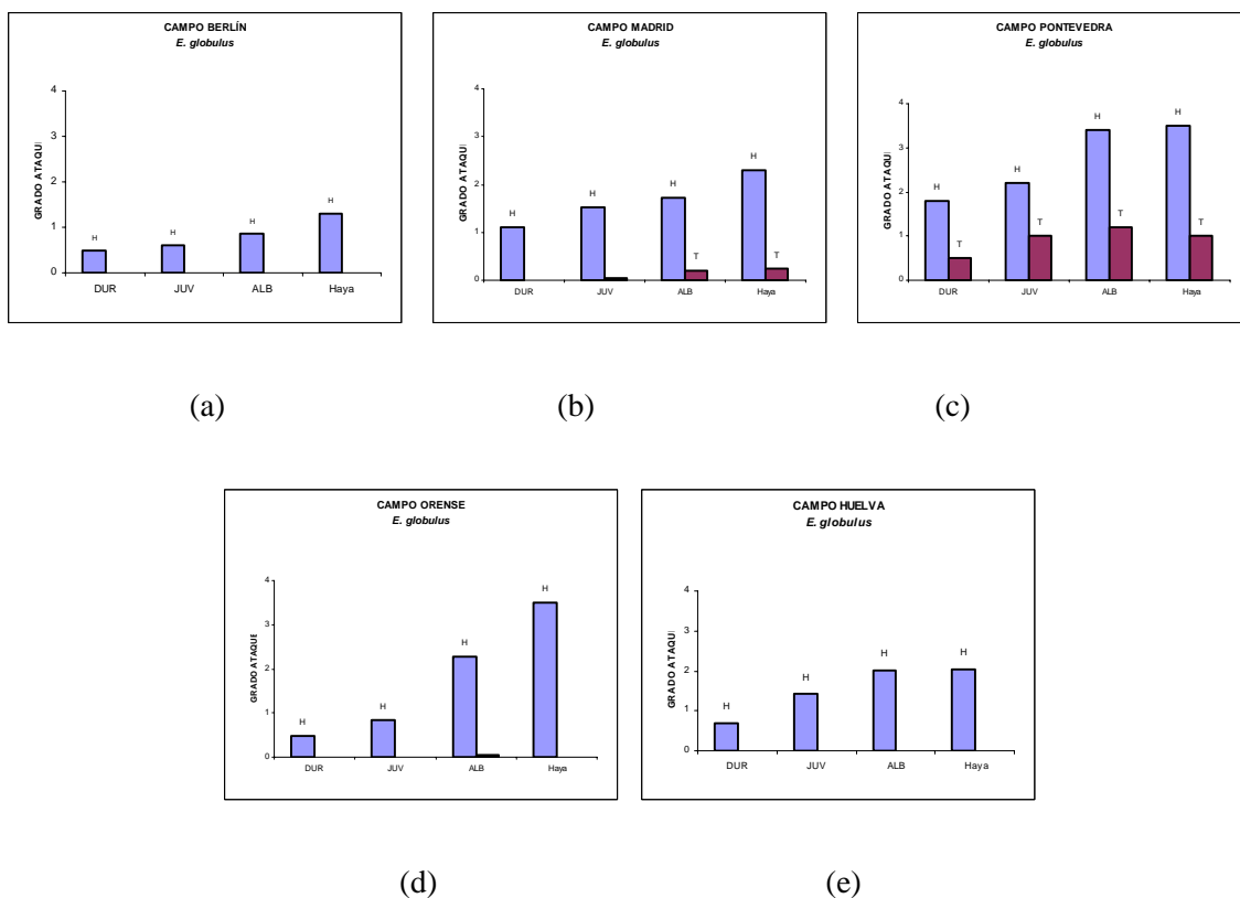
Fig. 2.- Valores medios de los grados de ataque producidos en la madera de albura (ALB), duramen (DUR) y juvenil (JUV), por los hongos xilófagos (H) y termitas (T) en los campos de ensayo de (a) Berlín, (b) Madrid, (c) Pontevedra, (d) Orense y (e) Huelva.
