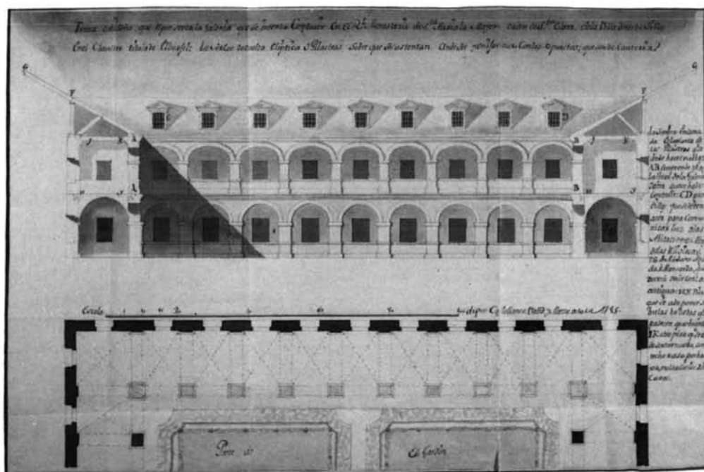
Tordesillas. Real Monasterio de Santa Clara. Claustro del Vergel. 1. Estado actual.— 2. Planta y alzado, por Francisco Pellón (1785). Archivo Histórico Nacional.
