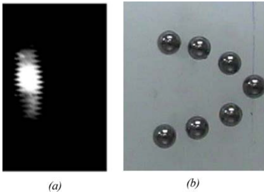
Fig. 5. (a) Representación en escala de grises de la imagen de 4 \times 8 \text{cm}^2 , debida al esparcimiento elástico de microondas evanescentes que viajan de izquierda a derecha hacia el arreglo parabólico de esparcidores sobre la superficie de parafina de un prisma; (b) la correspondiente imagen digital de la superficie (no está a escala).
