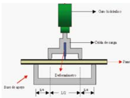
Figura 6a. Montaje del ensayo de corte en probetas
