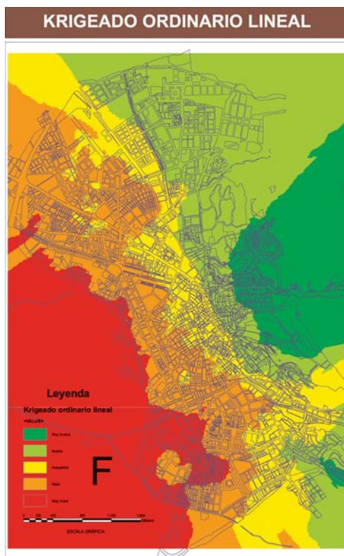
Figura 2. Microzonación sísmica obtenida a partir de la figura 1 tras aplicar krigeaje lineal ordinario
