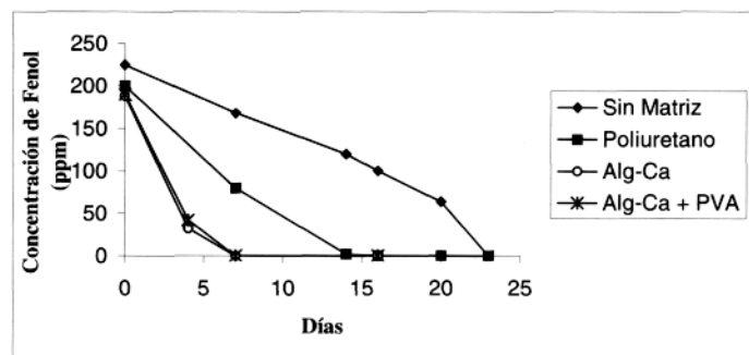
Figura 3. Comparación de las matrices en la remoción de fenol.
