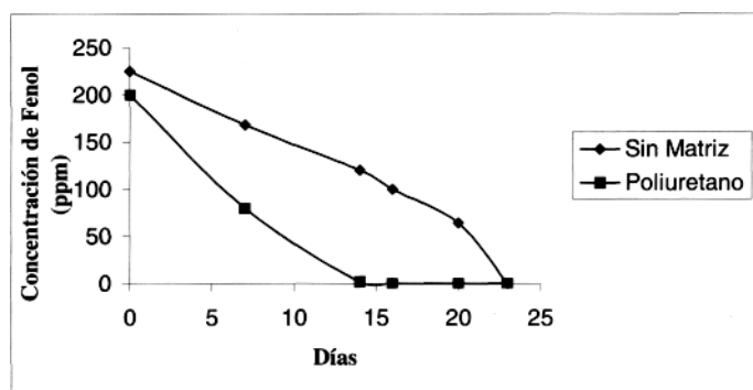
Figura 1. Degradación de Fenol en Matriz de Poliuretano
