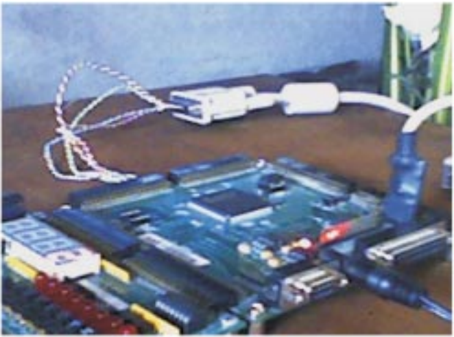
Figura 9. Prueba sobre la tarjeta Digilab DIO2
