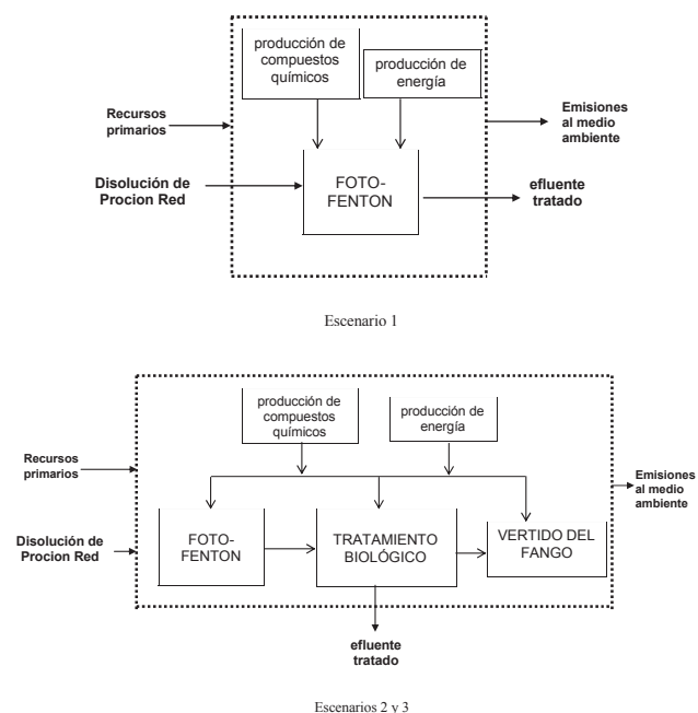
Figura 2. Diagrama de flujo de los sistemas correspondientes a los distintos escenarios
