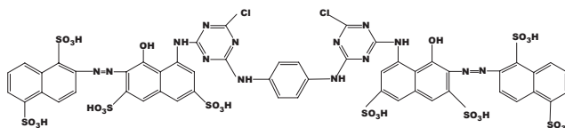
Figura 1. Fórmula molecular del colorante Procion Red H-E7B.
