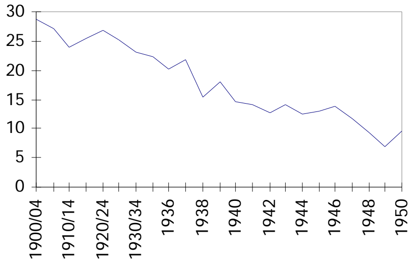
Gráfico 2.Evolución de las Importaciones y Exportaciones como porcentaje del PIB a coste de factores, 1900-1950 (precios constantes de 1950)
