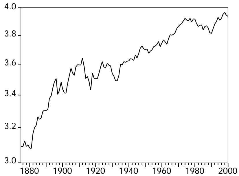
Gráfico 1. Serie de PIB per cápita Argentino, 1875-2000 (logaritmos)
