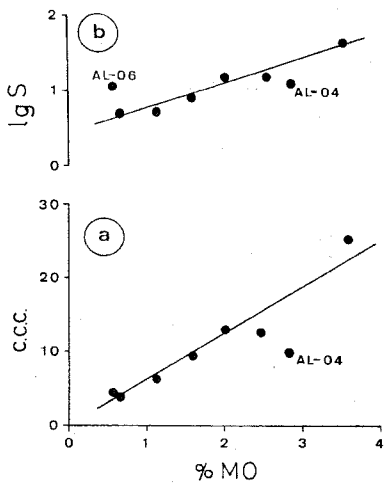
Figura 2.— Correlación entre la capacidad de cambio (a) y el logaritmo de la superficie específica (b) de los suelos con su contenido en materia orgánica.
