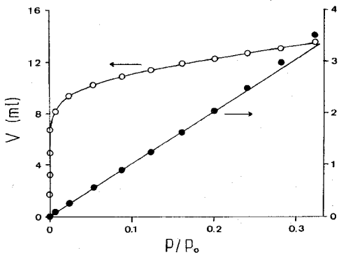
Figura 4.— Isotherma de adsorción de N_2 sobre el suelo AL-07 (○) y ajuste a la ecuación de B.E.T. (●).
