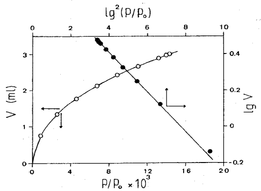
Figura 5.— Isotherma de adsorción de CO_2 sobre el suelo AL-07 (○) y ajuste a la ecuación de Dubinin (●).
