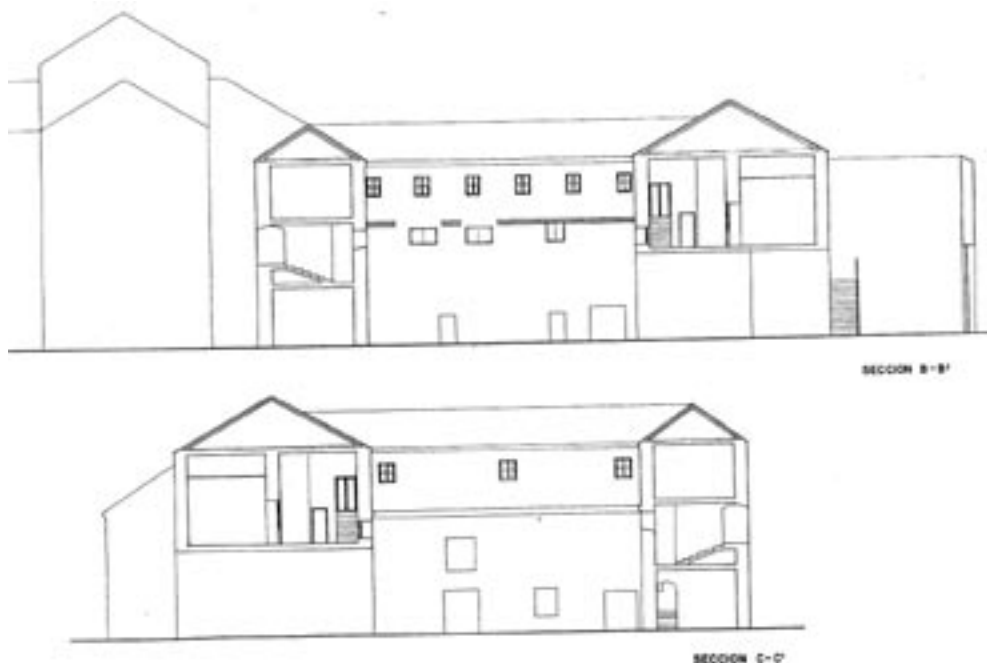
Sección del convento. Arqts. Demófilo Peláez y Nicolás Travési. Gerencia Municipal de Urbanismo.
