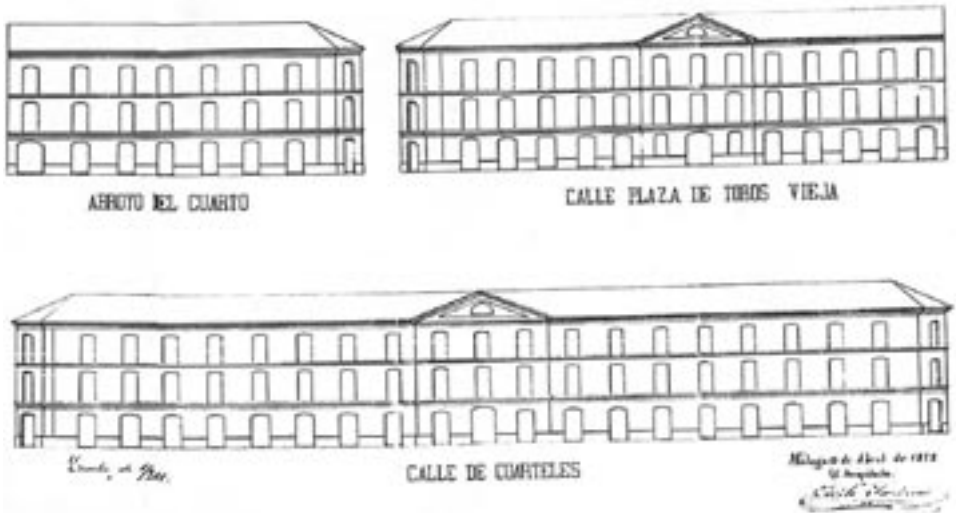
Proyecto de viviendas sobre el convento desamortizado. Arqto. Cirilo Salinas, 1872 (A.M.M.).
