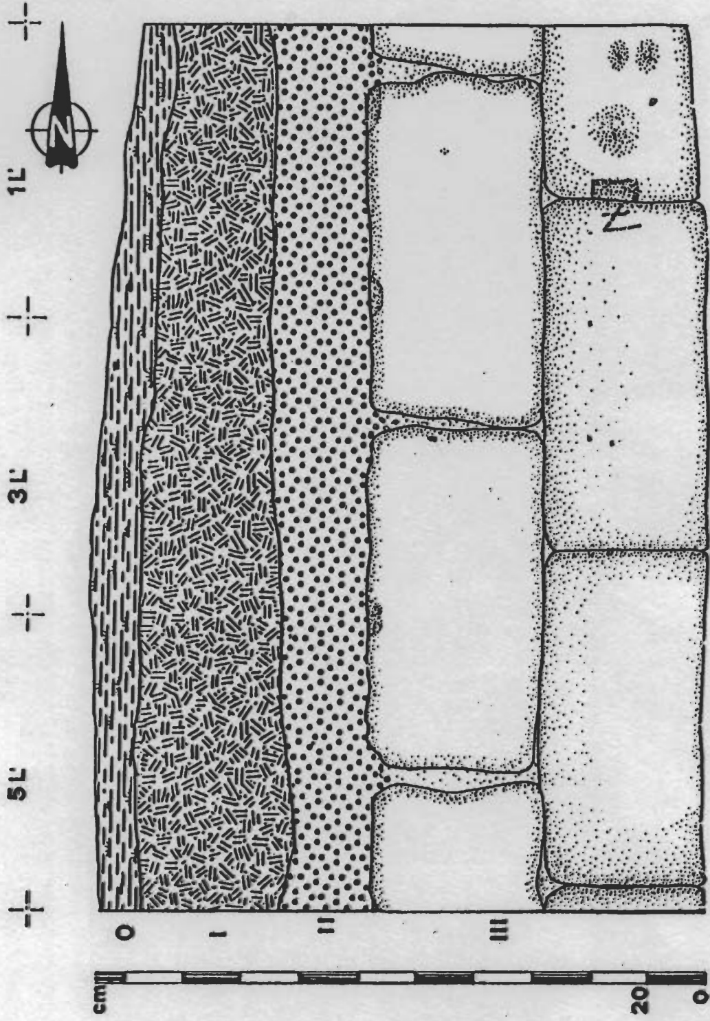
Lámina 11.—Corte estratigráfico de ladera este.
