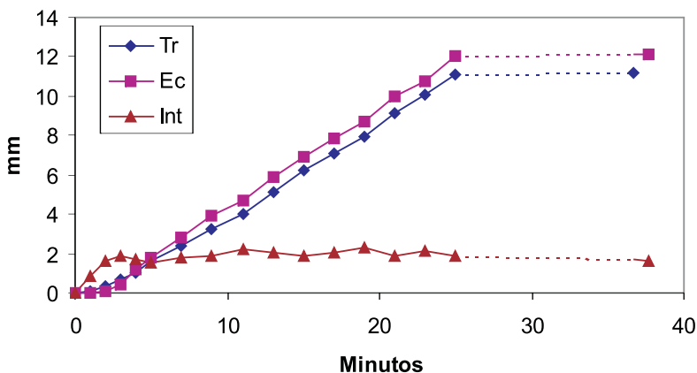
FIGURA 3. Hidrograma completo de los valores acumulados de trascolación (Tr), escorrentía cortical (Ec) e interceptación (Int) en tomillo (promedio de las tres simulaciones).
